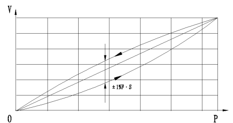
典型静态校准误差曲线
